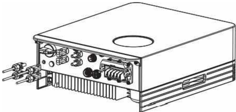
▲ Рисунок 4.12 Подключите разъем постоянного тока к инвертору
