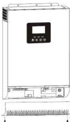
Рисунок 6 Установка защитной крышки
