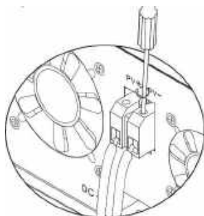
Рисунок 5 Подключение кабеля солнечных панелей
