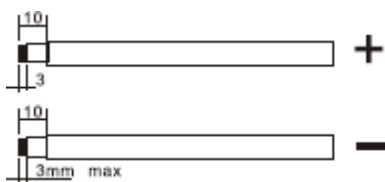
Рисунок 4 Разделка солнечного кабеля
