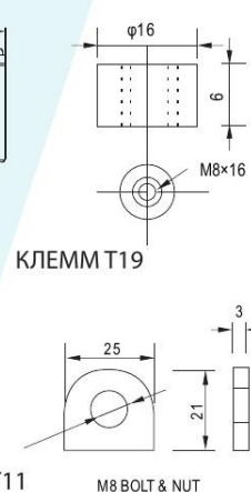
ТИП КЛЕММ
